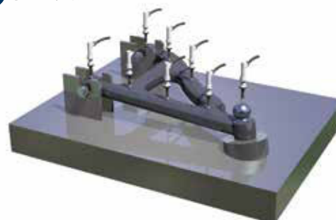
⑧ 检测夹具
